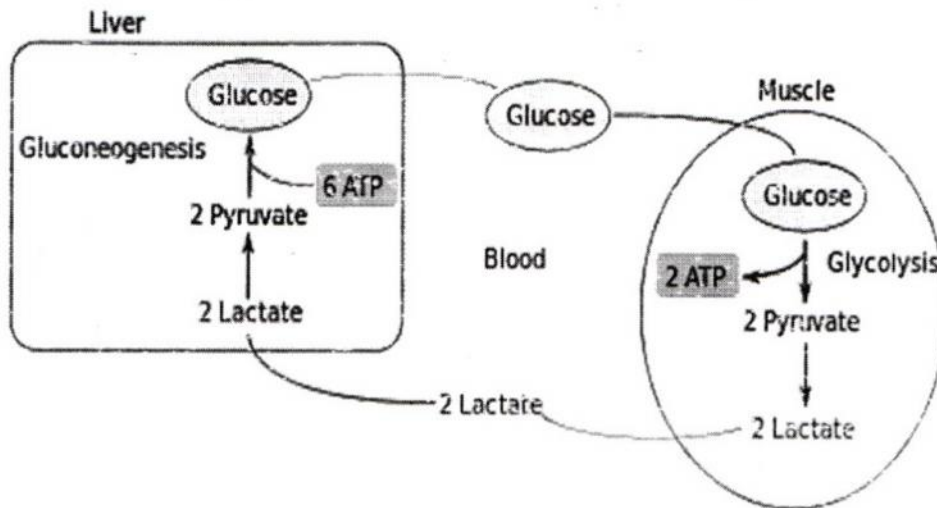
Gambar 2.7 Siklus Cori
